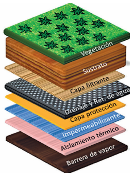
Figura 1. Composición de un techo verde. Fuente: Morales, Cristancho & Baquero [12]
